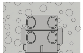
Betondecke mit tiefer Schalterdecke (Schraubabstand 60mm)
